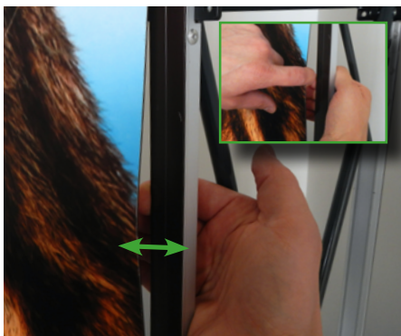
16 Paneelen von hinten lösen und Bildübergänge ausrichten.
