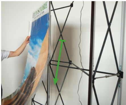
13 Schutzhülle langsam nach unten ziehen. Paneele bleibt am System.
