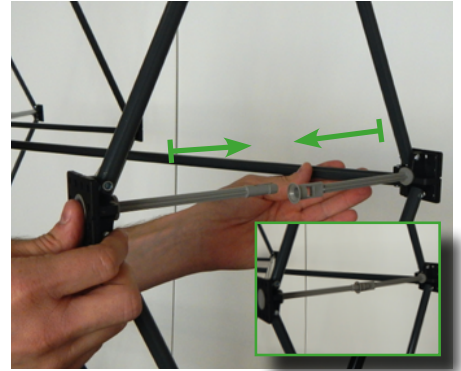
3 Kunststoffverriegelungen zusammenklicken.
